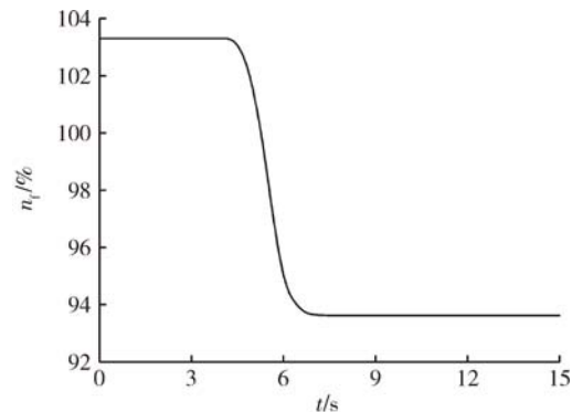
(b) 风扇转速 n_t 变化
