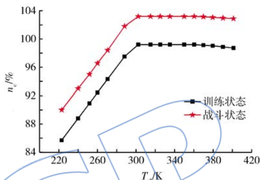
图 5 中间状态 n_c 和 T_{12} 函数关系
