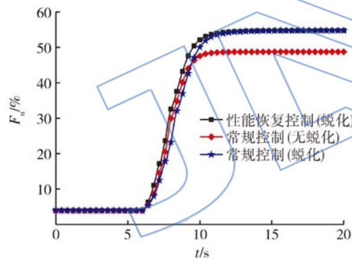
(c) 推力 F_n 比较
