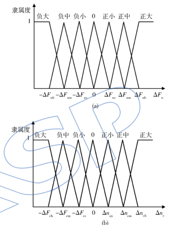
图 3 输入与输出的隶属度函数
