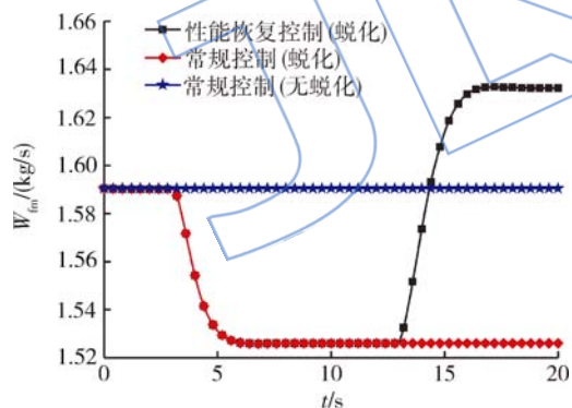
(a) 主燃油流量 W_{fm} 比较
