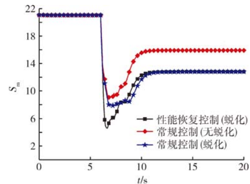
(d) 喘振裕度 S_m 比较
