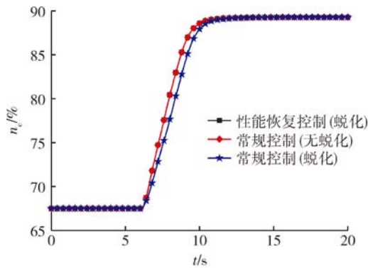
(b) 压气机转速 n_c 比较
