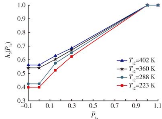
图 15 不同 T_{t2} 下的 h_2(\bar{P}_{la}) 函数关系曲线
