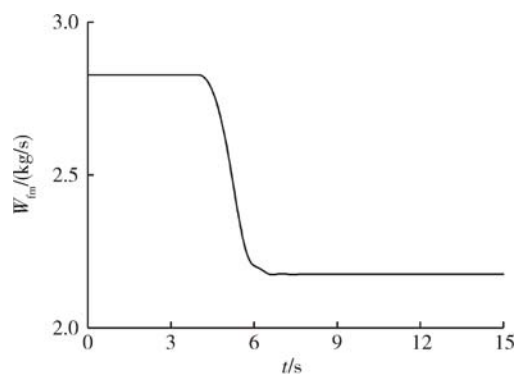
(a) 主燃油流量 W_{fm} 变化
