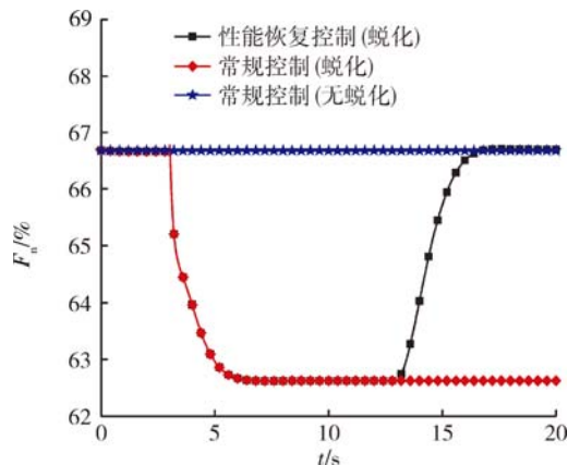
(c) 推力 F_n 比较
